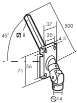
SORTIE CAISSON 45° P/AXE 4 TROUS.
