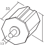
EMBOUT EN PLASTIQUE P-12
